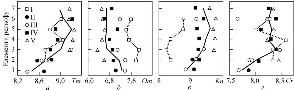
Рис. 3.20. Значення режимів кліматичних факторів (в балах) для рослинних угруповань різних форм рельєфу в степовій зоні:
