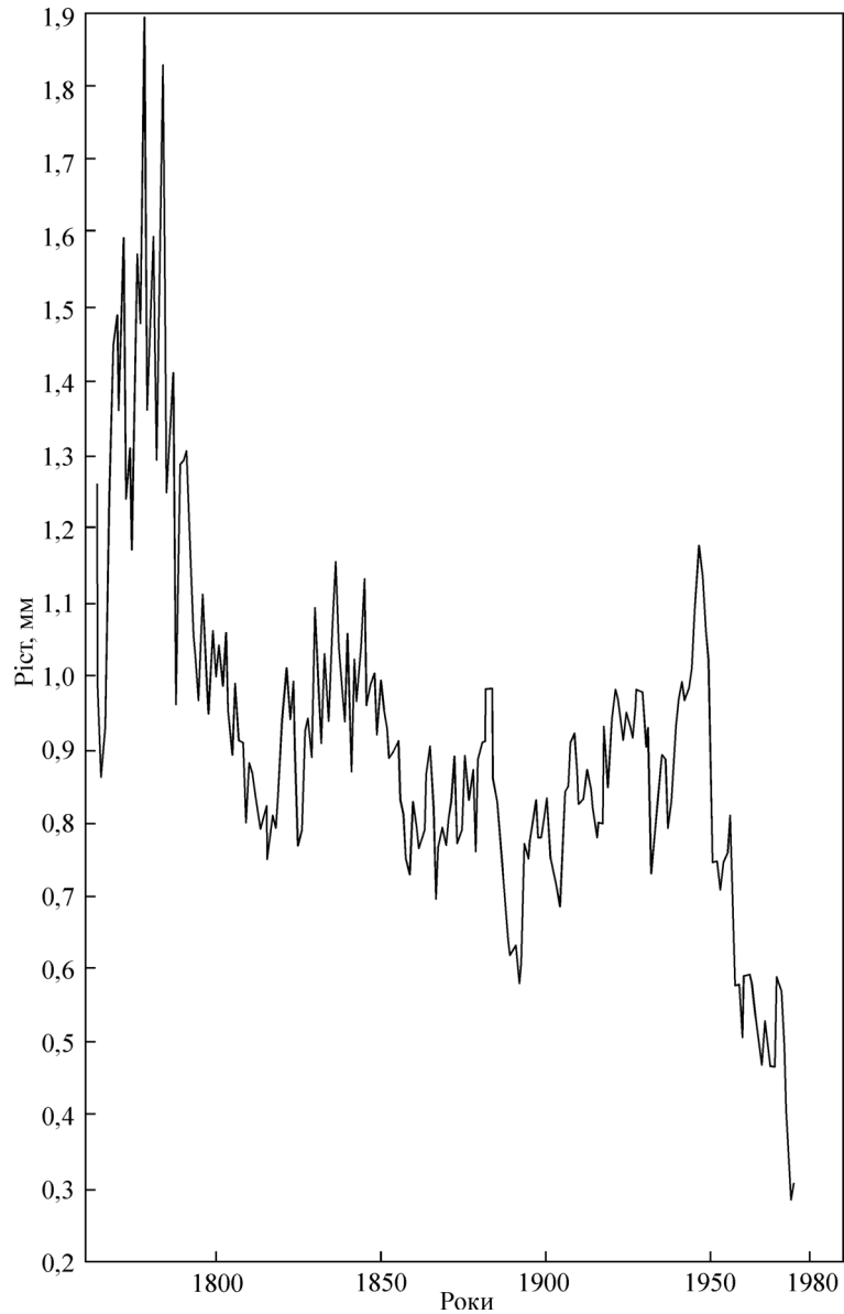
Рис. 1.19. Дендродіаграма росту річних кілець Pinus sylvestris у зоні забруднення викидами деревообробних підприємств у м. Братськ (Lovelius, 1997)
