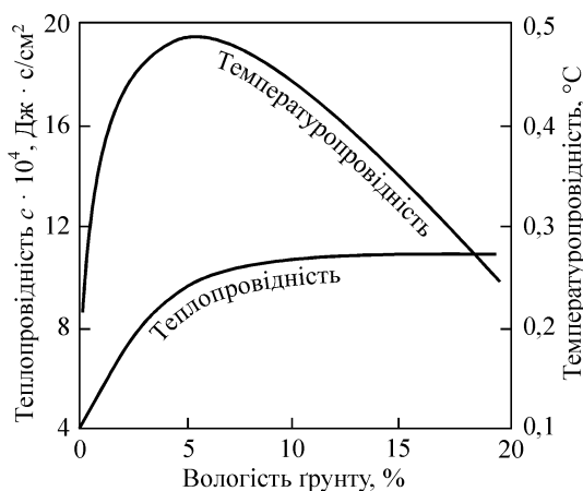
Рис. 2.10. Залежність між показниками вологості, теплопровідності й температуропровідності різних типів ґрунтів
