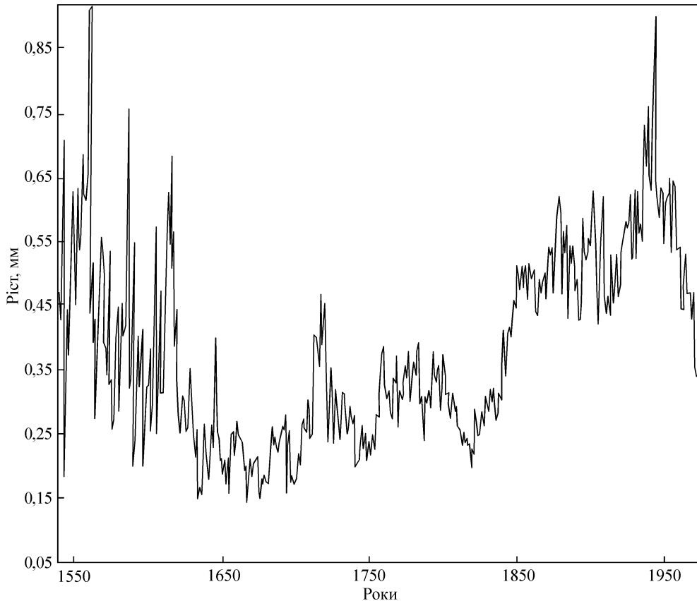
Рис. 1.17. Фрагмент узагальноної дендрограми, створеної на основі середніх значень росту хвойних у 10 північних регіонах Євразії (Lovelius, 1997)
