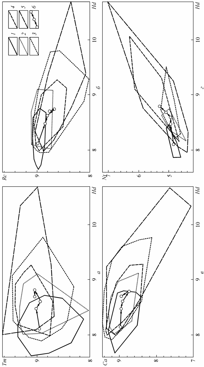
Рис. 3.33. Загальні зміни екострою рослинних угруповань абсолютно запівідної ділянки «Хомутівський степ» з 1969 по 2005 р., отримані за методикою синфітоіндикації (Гкаченко, 2008)
