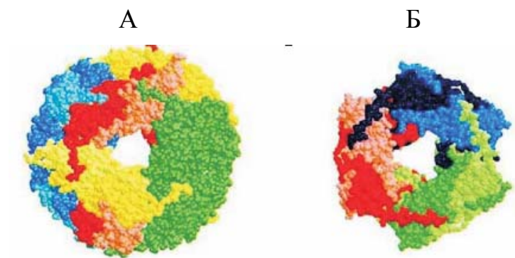
Рис. 3. Структура олигомеров нмБТШ 16,5 Methanococcus jannaschii (А) и БТШ 16,9 Triticum aestivum L. (Б)
